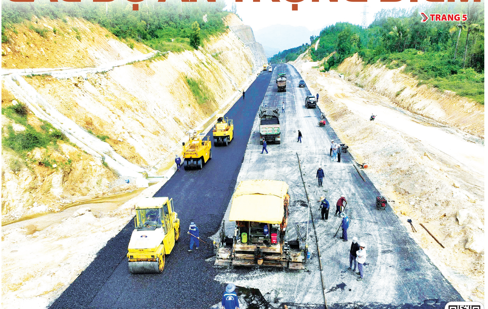
Dự án Cao tốc Bắc - Nam đoạn qua địa bàn tỉnh Đắk Lắk đang dần được đầu tư hoàn chỉnh. Ảnh: Thanh Xuân
